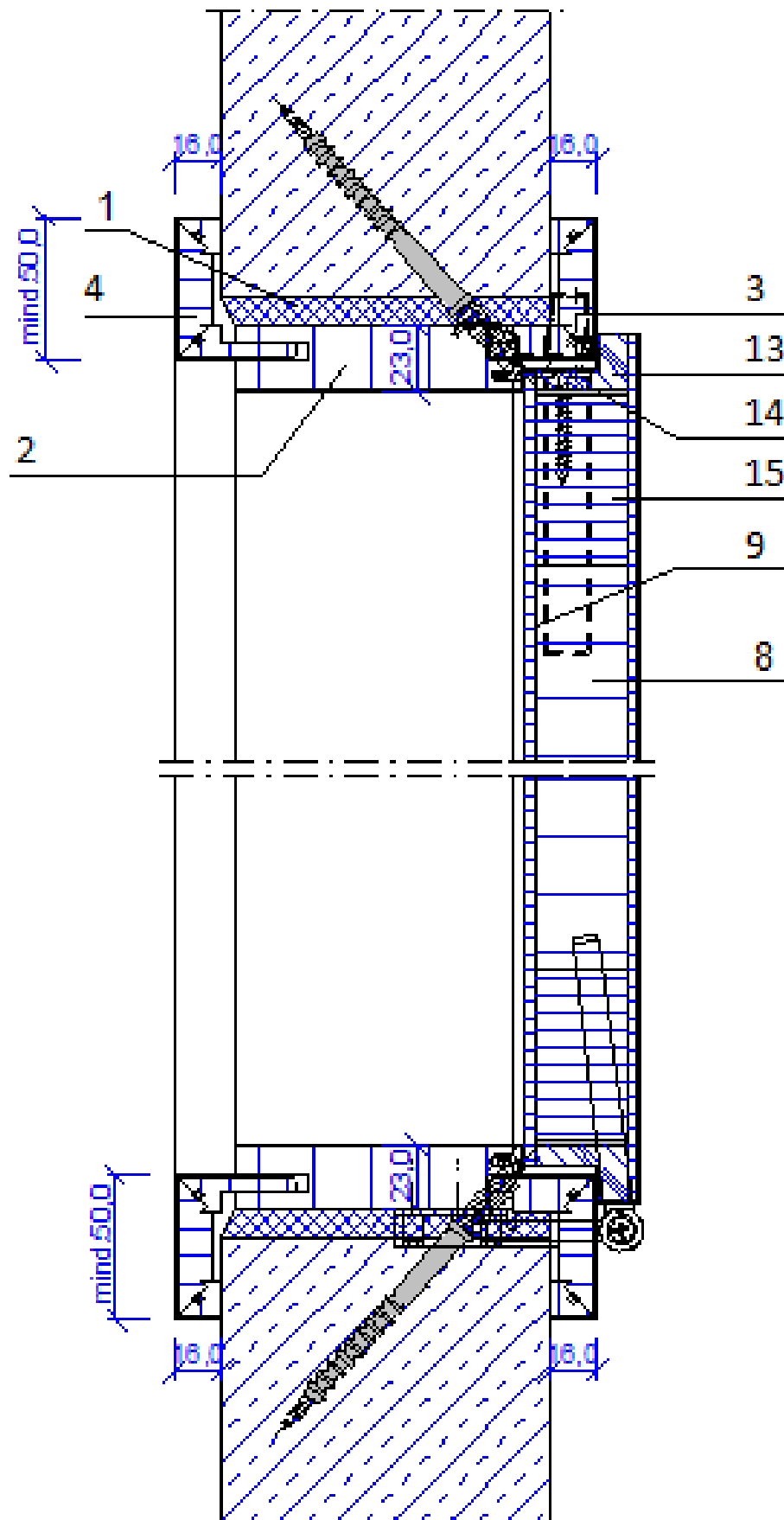
Figuur 4 - Horizontale snede - Type B
