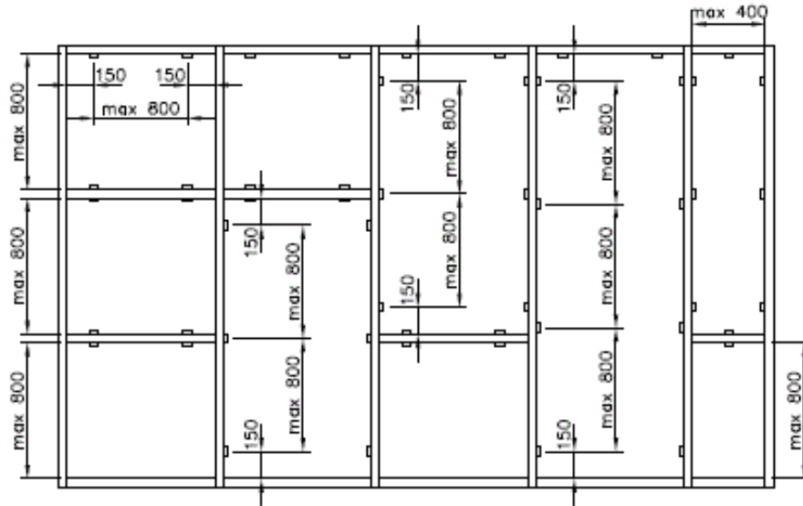
Fig 7b: Aantal en plaats glasklipsen (max. glashoogte 2300 mm)
