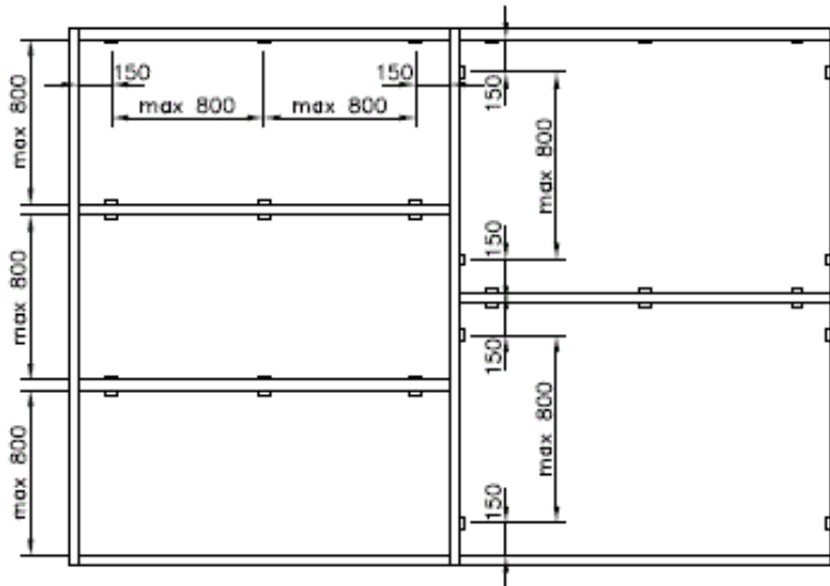
Fig 7c: Aantal en plaats glasklipsen (glashoogte > 2300 mm)
