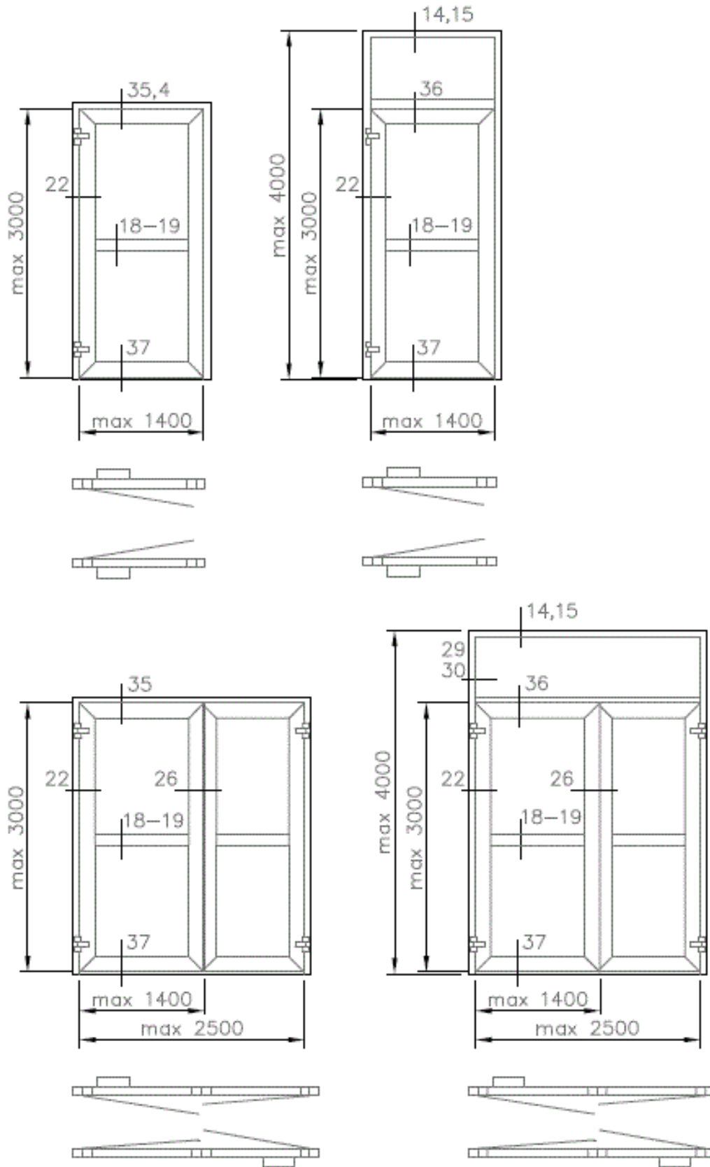
Fig. 1b: Ensembles de portes résistant au feu EI 30 (74421)
